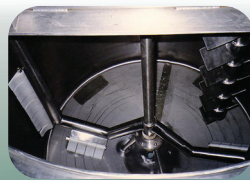
• AGITATOR
